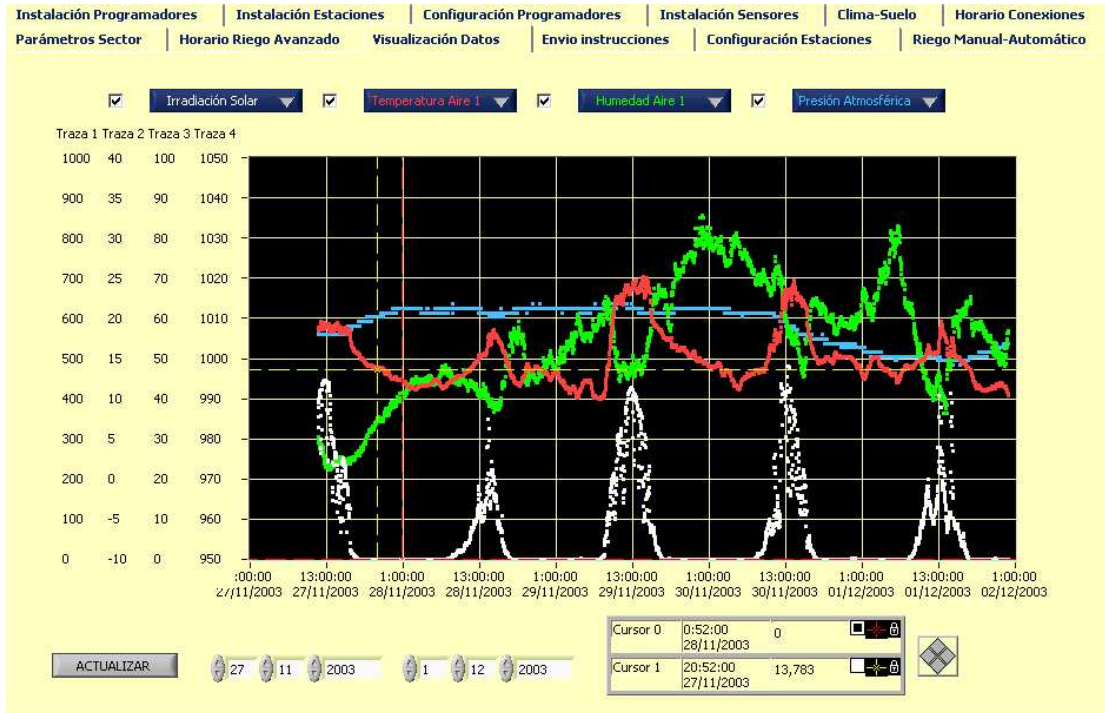
Fig.26. Histórico de los registros de datos clima-suelo
